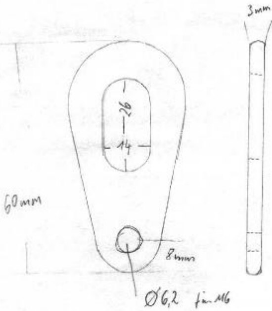
Platte
